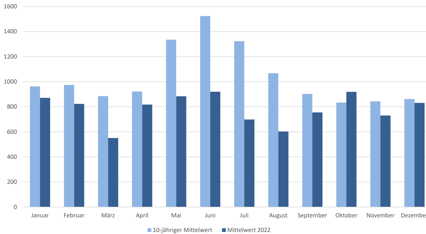
Tagesmittelwerte des Abflusses am Pegel Rheinfelden 2022
